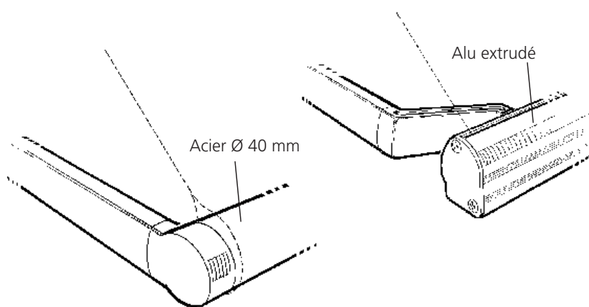
FIXATION BRAS SUR BARRE DE CHARGE
