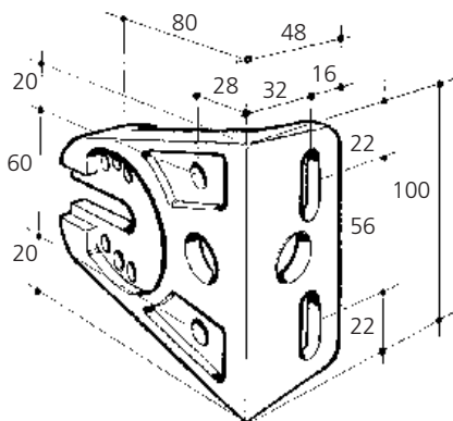
FIXATION BRAS SUR BARRE DE CHARGE
