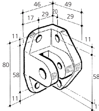
CHAPPE DE BRAS STANDARD
