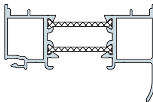
Élargisseur 25 mm - aile 15 mm
