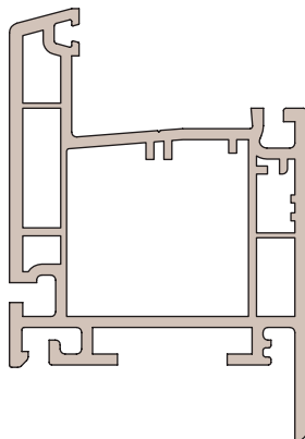
Dormant aile 40
