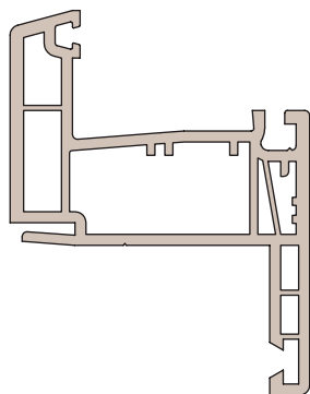
Dormant aile 30
