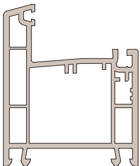
Dormant base
