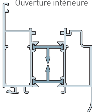
Dormant doublage (tapée + aile 15)
