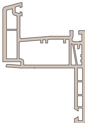
Dormant aile 40
