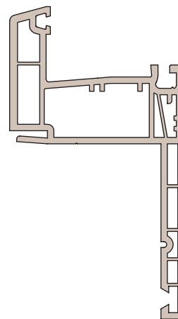
Dormant aile 60
