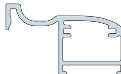
Couvre joint ALU 35x20 - mouluré
