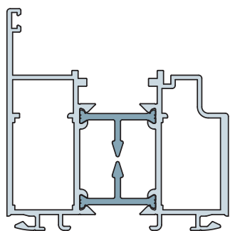
Dormant double gorge
