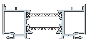
Élargisseur 25 mm - sans aile
