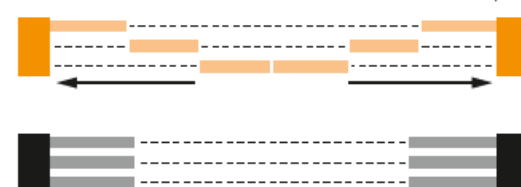
6 vantaux sur 3 rails - ouverture 2/3
